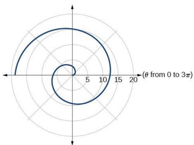
27. Archimedes' spiral
