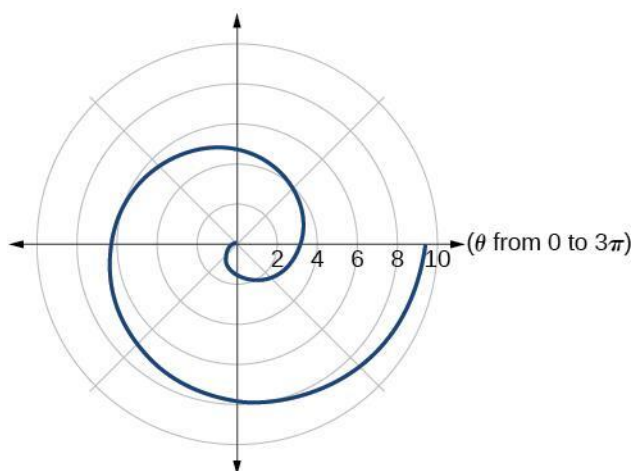
27. Archimedes' spiral
