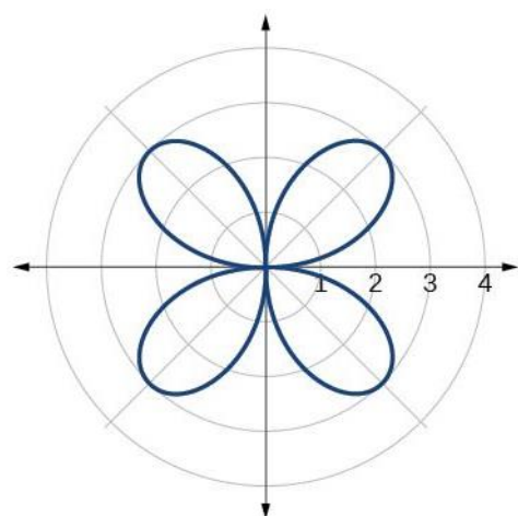
21. Rose
