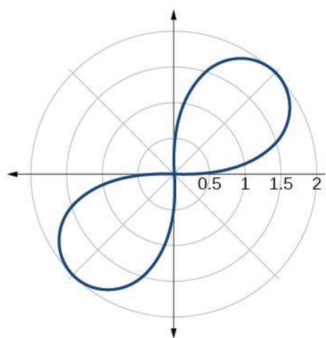
19. lemniscate
