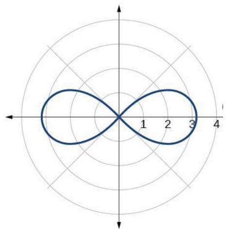
18. lemniscate
