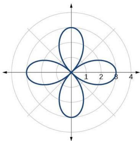
23. Rose
