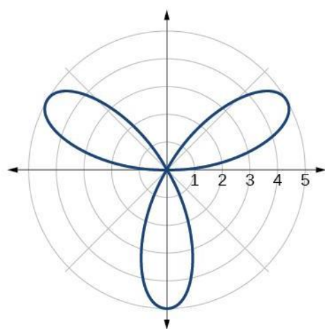
24. Rose
