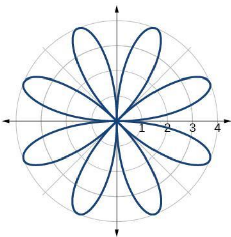
24. Rose
